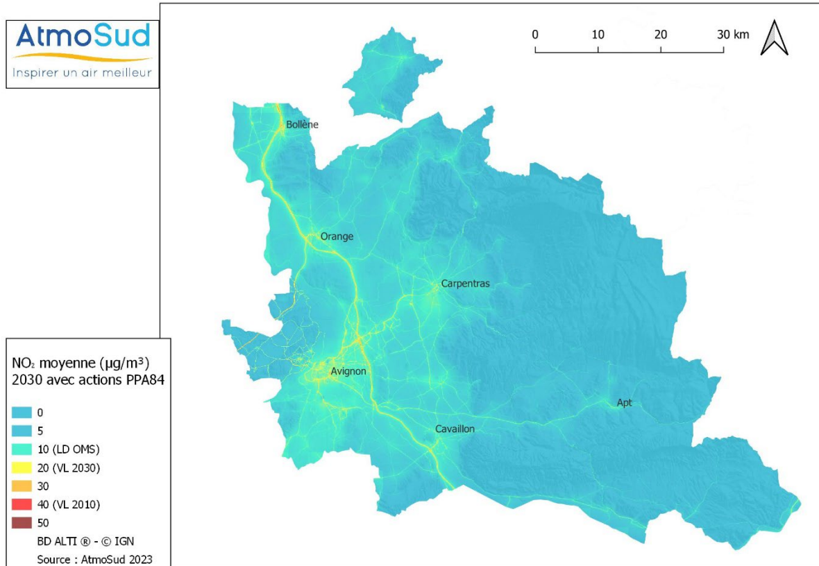
Figure 26 : Carte des concentrations des moyennes annuelles en \text{NO}_2 à l'échelle du PPA 84 pour l'année 2030 avec la prise en compte du tendanciel et des actions du PPA
