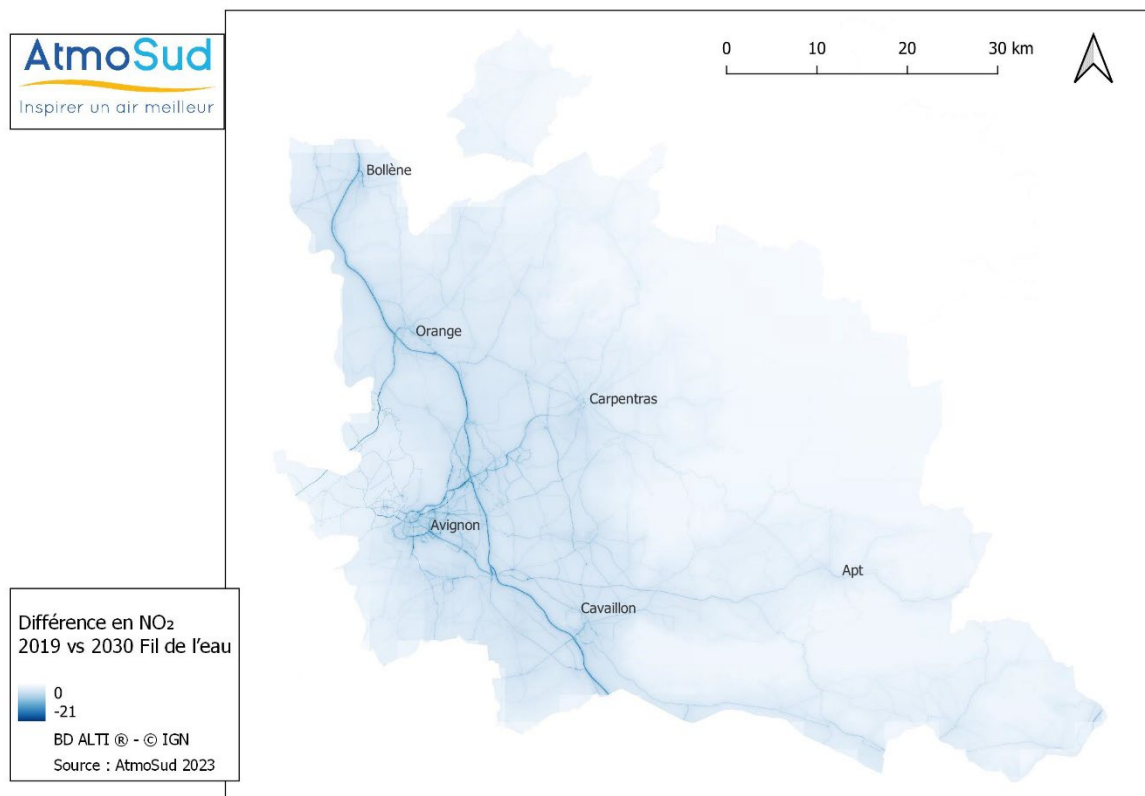
Figure 27 : Carte des différences des concentrations des moyennes annuelles en \text{NO}_2 à l'échelle du PPA 84 entre l'année 2030 avec la prise en compte du tendanciel et des actions du PPA et l'année 2019
